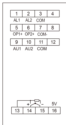
D71 接线图
