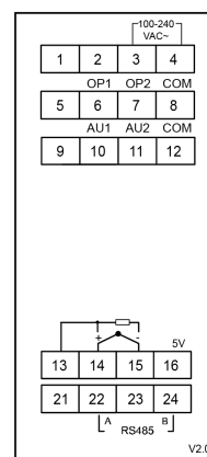
E7 接线
