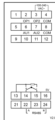
E7接线图
