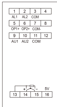
新D71接线图
