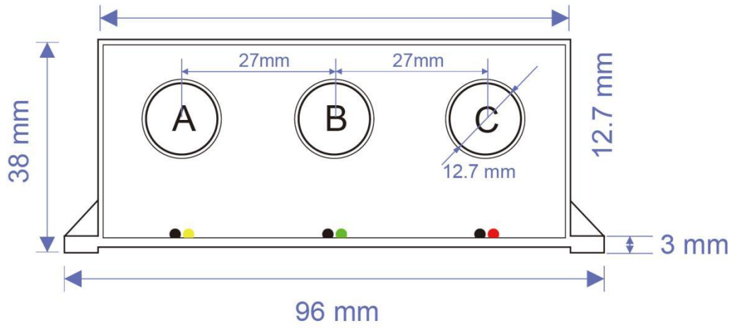
主视图
